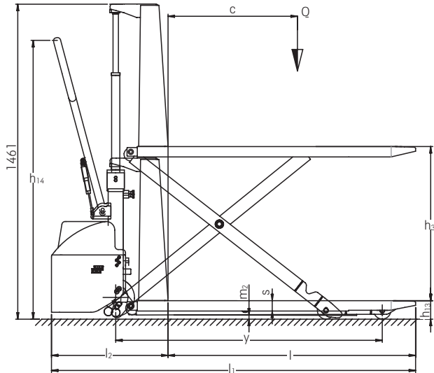
HPT 10 XE Vista lateral
