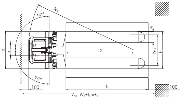
HPT 10 XE Vista superior
